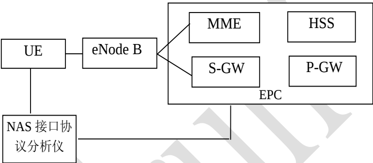
图 1 终端与核心网测试环境示意
